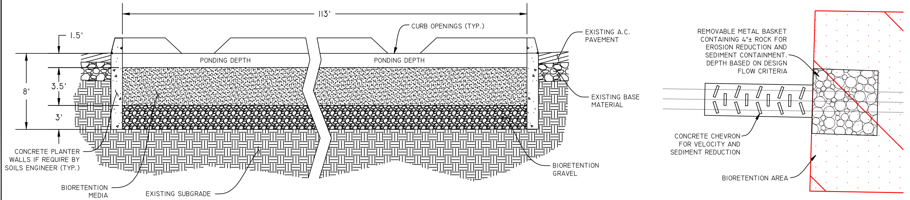
SECTION A-A
